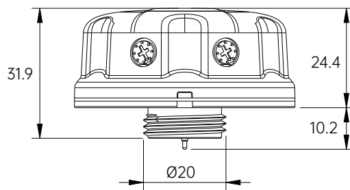
HD09VR-MH/HD09VR-MHB
