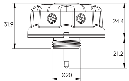
HD09VR-MH-1/HD09VR-MHB-1
